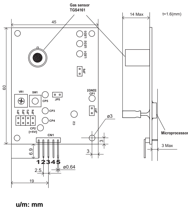
Fig. 1 - CDM4161 dimensions
